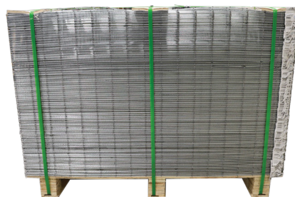
Art.nr 115812 Armeringsnetting galvanisert stål 120 cm x 80 cm, tykkelse 2,5 mm (300)
